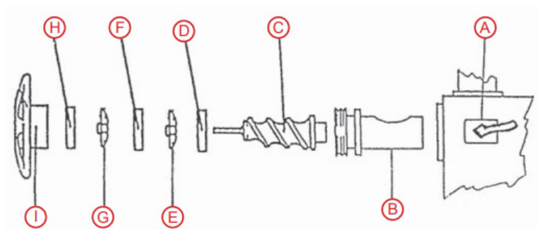
Obr. 2 Rozebírka dvousložení neodnímatelná hlava
